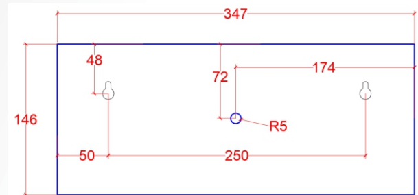
Kích thước mặt sau bảng báo cháy
